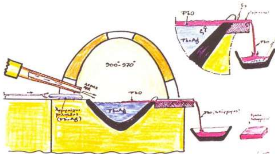
Τομή της καμίνου για την Κυπέλλωση του αργυρούχου μολύβδου, κατά τον Κ. Κονοφάγο.
